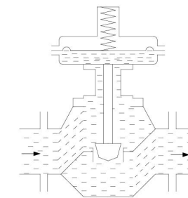
自力式阀前微压调节阀的工作原理图
