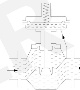
自力式阀后微压调节阀的工作原理图
