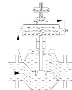
带指挥器操作自力式阀前调节阀 工作原理图
